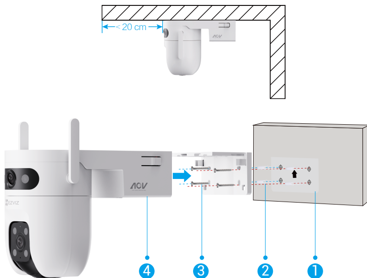
Fig. 2 Veggmontering
